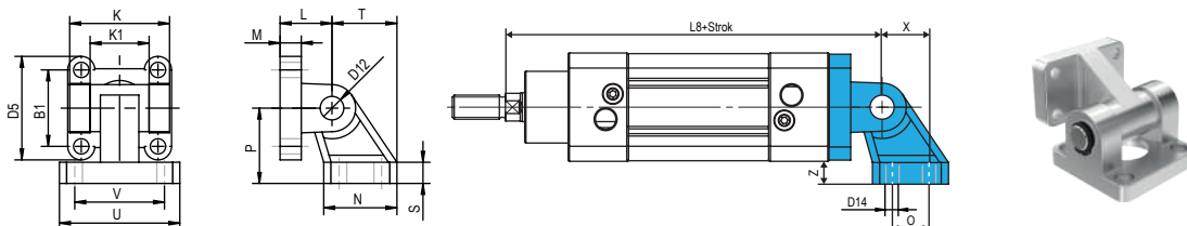
Серия ISO
